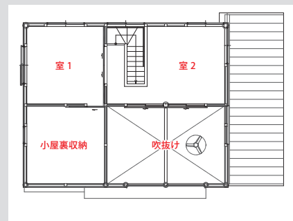
2F 平面図
